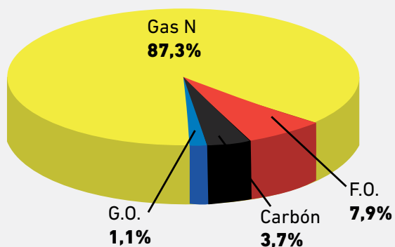
Consumo de Combustibles Fósiles Abril 2017
